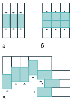
Однорядная (а), двухрядная (б) и кластерная (в) блокировка
