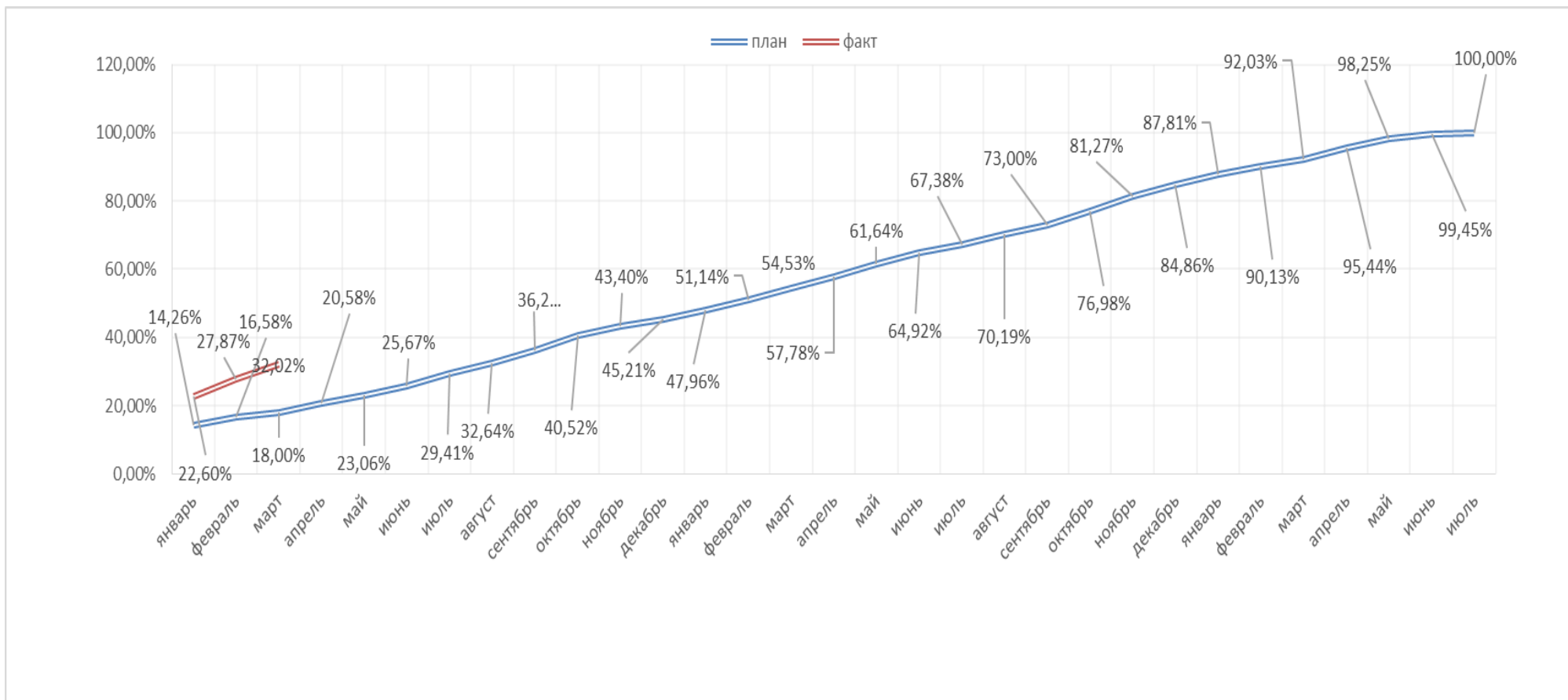
График Работ Производства (ГПР) начало 12 июля 2021 года - окончание 01 июля 2024 года Процент фактического выполнения вычислен согласно ЗКС и АВР.
